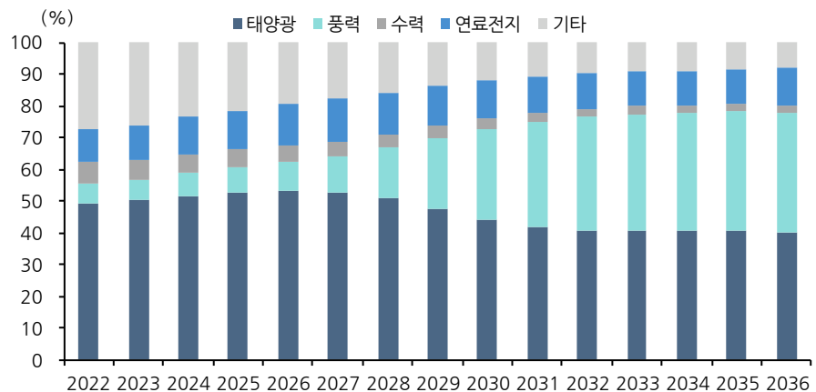
그림 30. 신재생 에너지원 발전량 믹스
