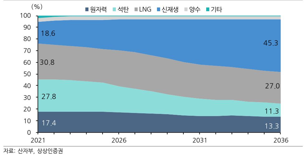
그림 8. 제10차전력수급기본계획, 전원 비중 전망
