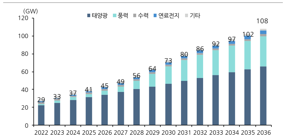
그림 7. 제10차전력수급기본계획, 신재생에너지 설치량 전망
