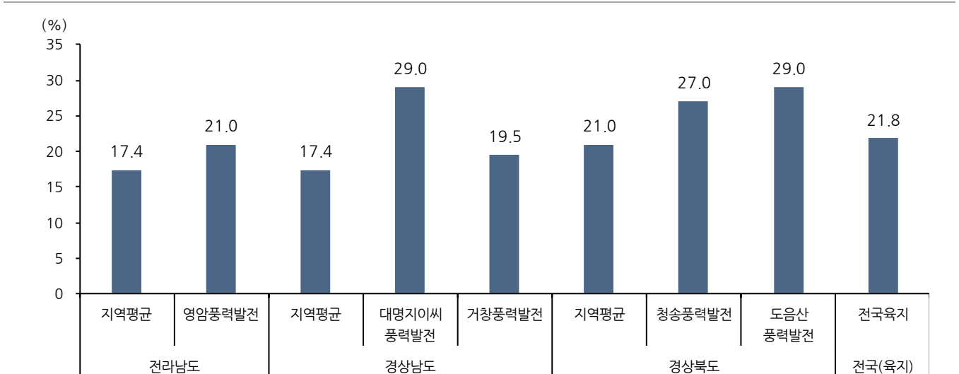
그림 7. 대명에너지 Micro-Siting 사업 vs 해당 지역 평균 이용률 비교
