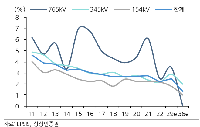
그림 23. 변전 설비 용량(MVA 기준)_7년 CAGR 증가율.
