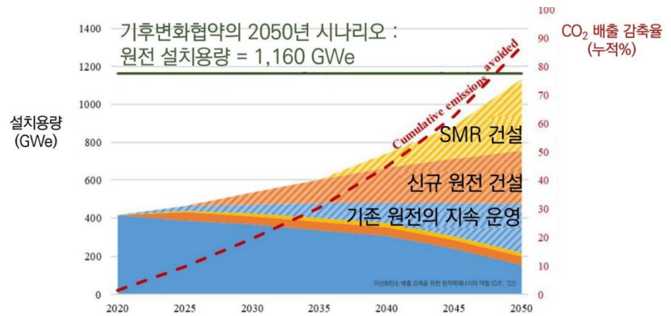
그림 15. 온실가스 배출 감축을 위한 원자력 설치 필요 용량
