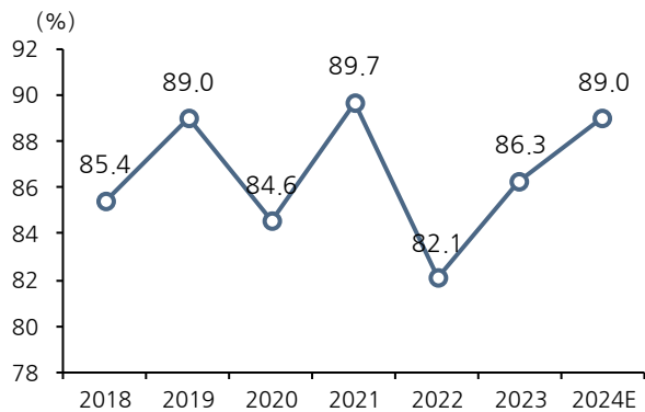
그림 7. 연간 발전소 가동률 추이
