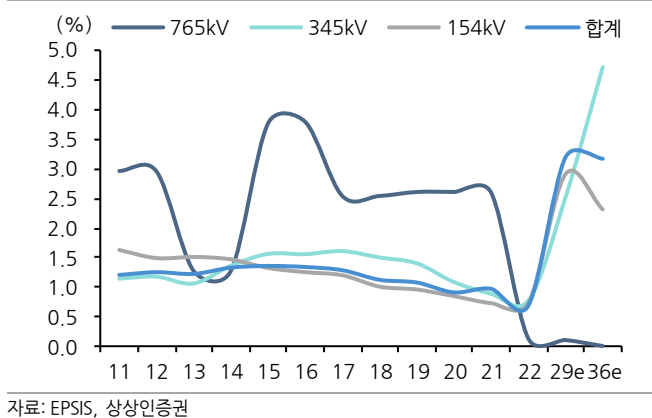
그림 22. 송전 선로 길이(C-km)_7년 CAGR 증가율.
